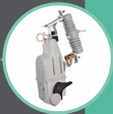
Religador Montado em Chave Fusível TripSaver® II
