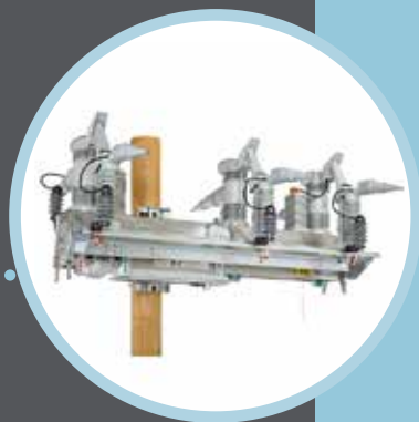
Interruptor de Faltas IntelliRupter® PulseCloser®
